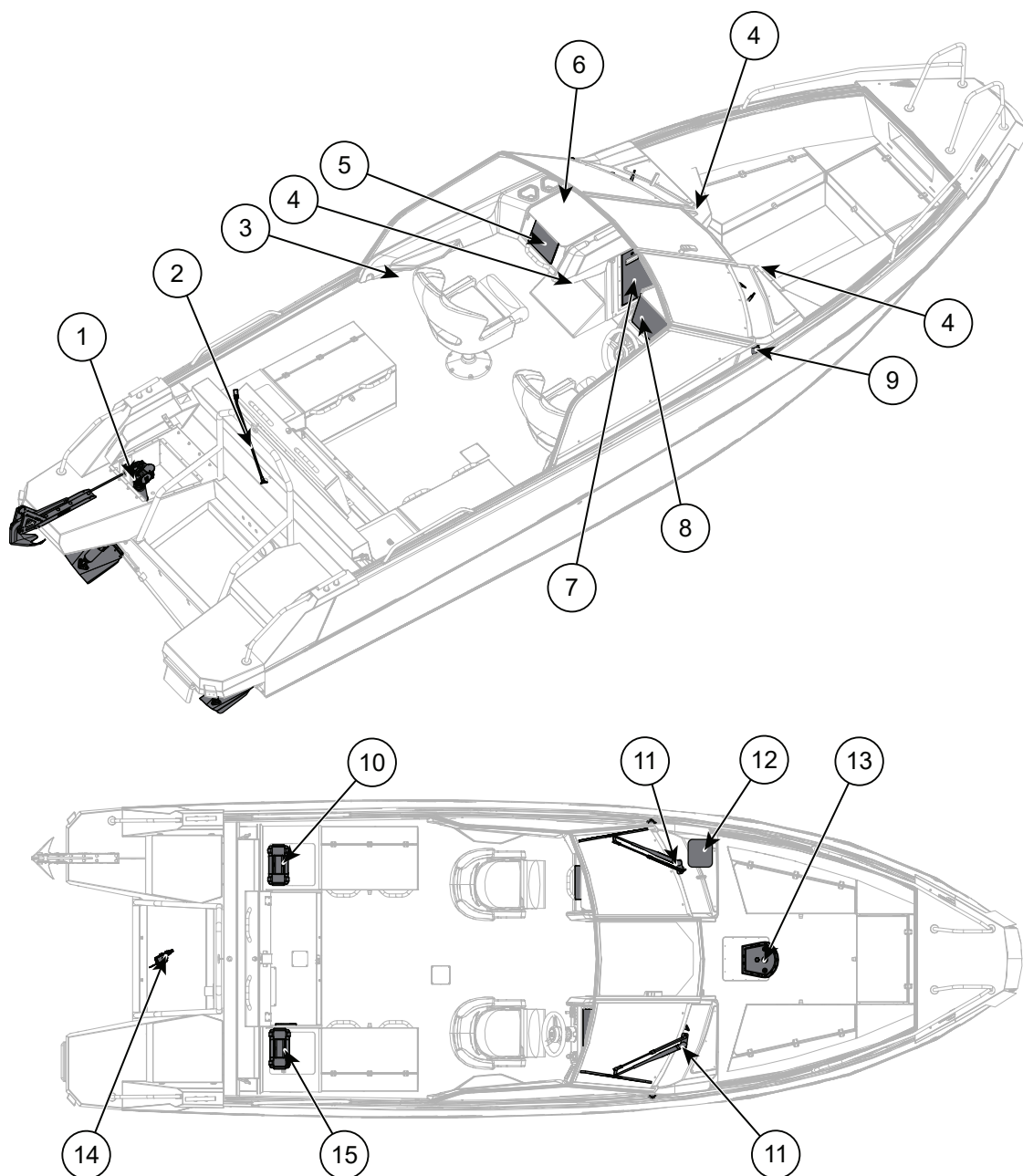
Figur 8.3 Buster Magnum/SuperMagnum elektrisk utstyr
