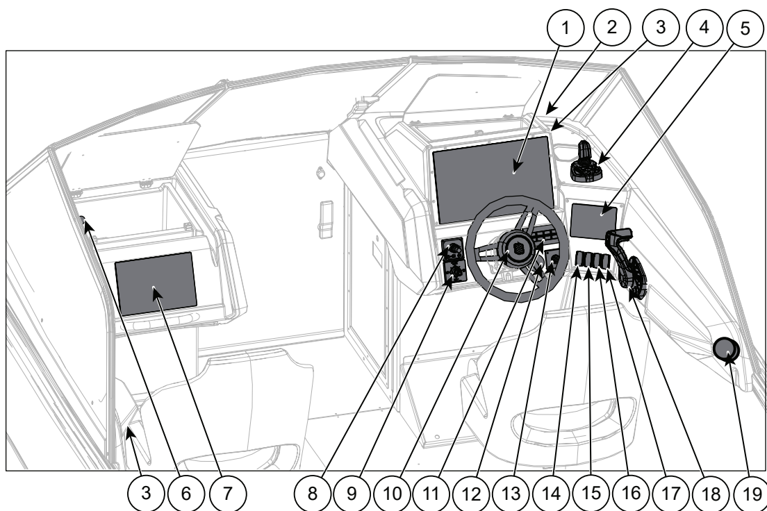
Figur 5.1 Buster Magnum/SuperMagnum styrestasjonskontroller
