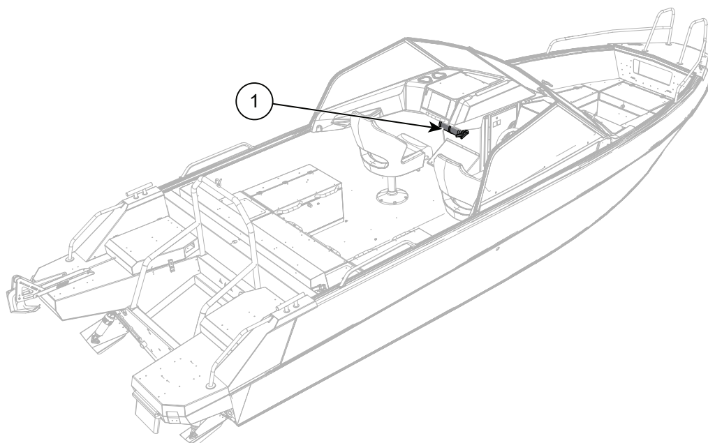
Figur 2.2 Buster Magnum/SuperMagnum plassering av brannslukningsapparat
