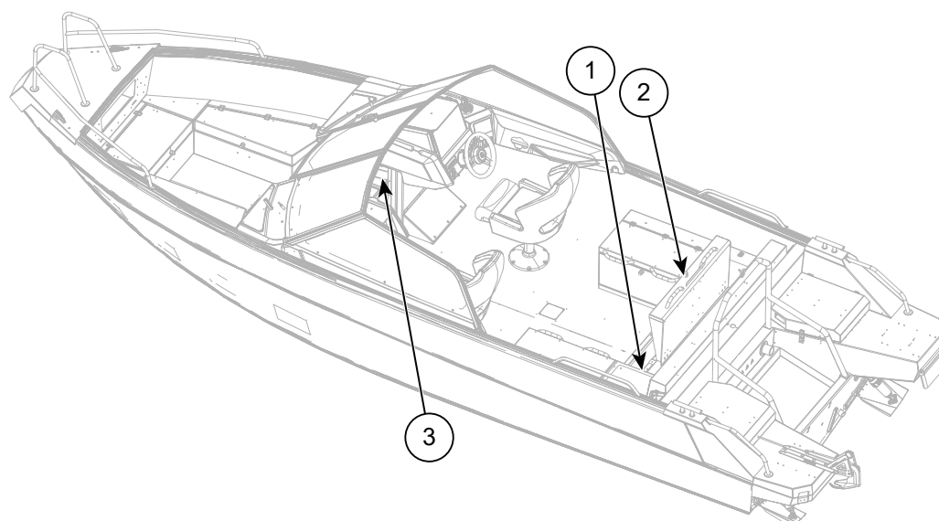
Figur 8.2 Buster Magnum/SuperMagnum plasseringer av sikringspanel
