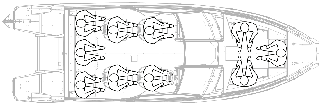
Figur 4.3 SuperMagnum performance-pakkeseter for maksimalt ti (10) passasjerer
