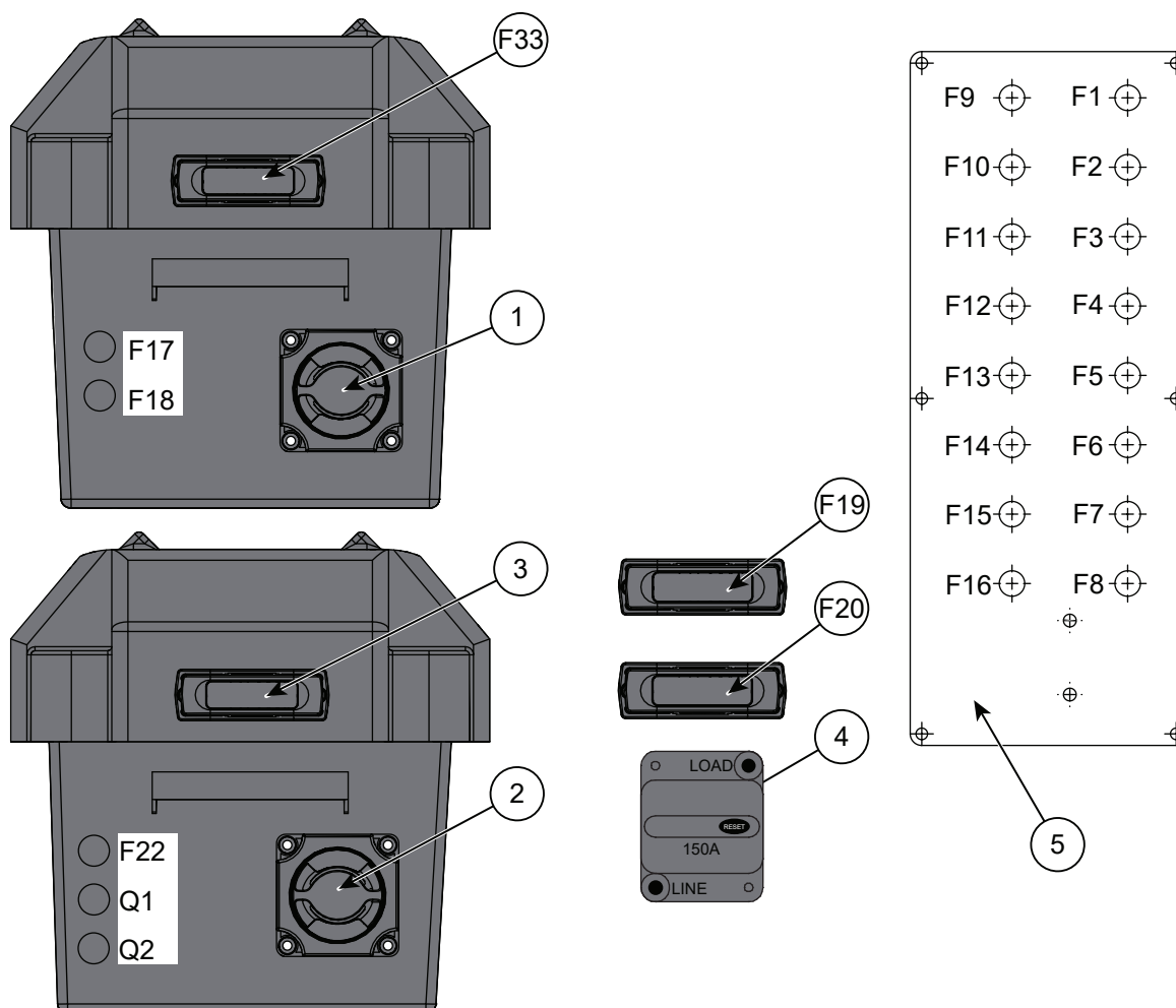
Figur 8.1 Buster Magnum/SuperMagnum hovedbrytere og sikringspaneler
