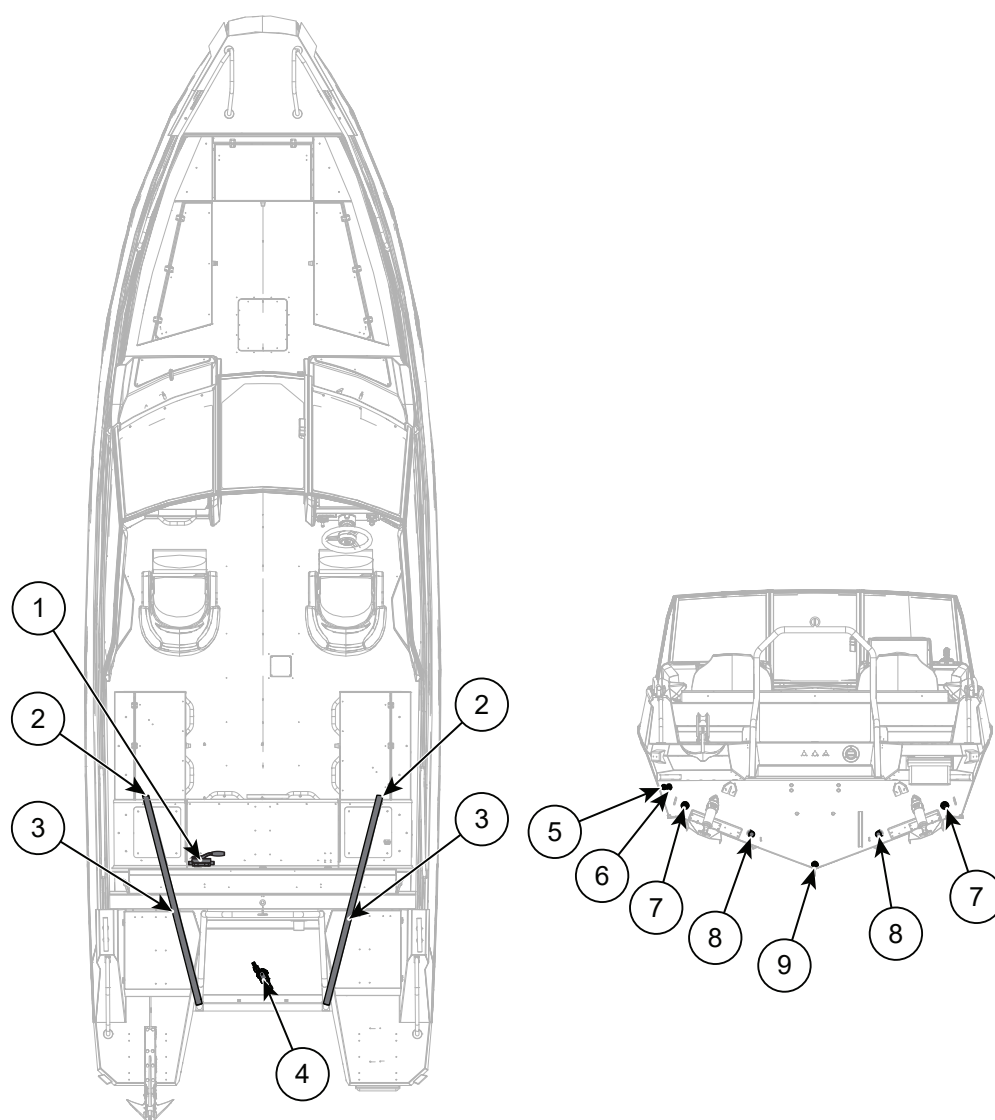
Figur 9.1 Buster Magnum/SuperMagnum lensepumper og drenering
