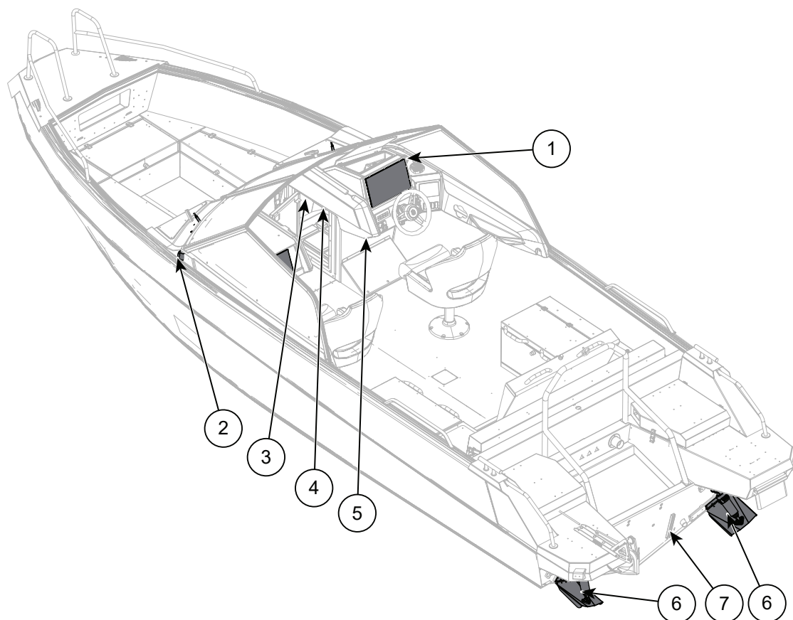
Figur 8.4 Buster Magnum/SuperMagnum elektrisk utstyr
