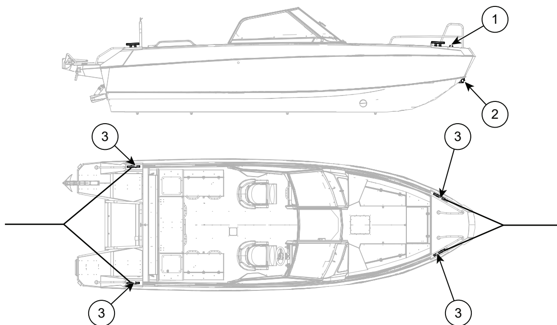
Figur 5.11 Buster Magnum/SuperMagnum fortøynings- og slepepunkter
